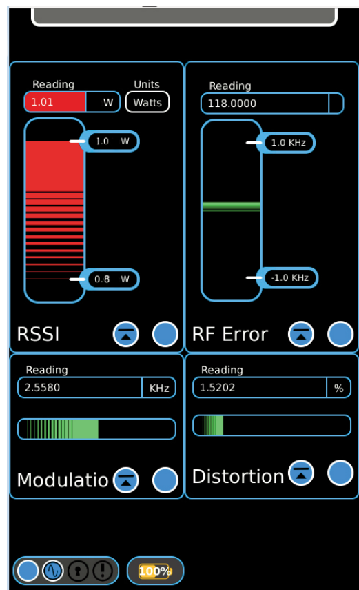
The 3550 Meter Formats
